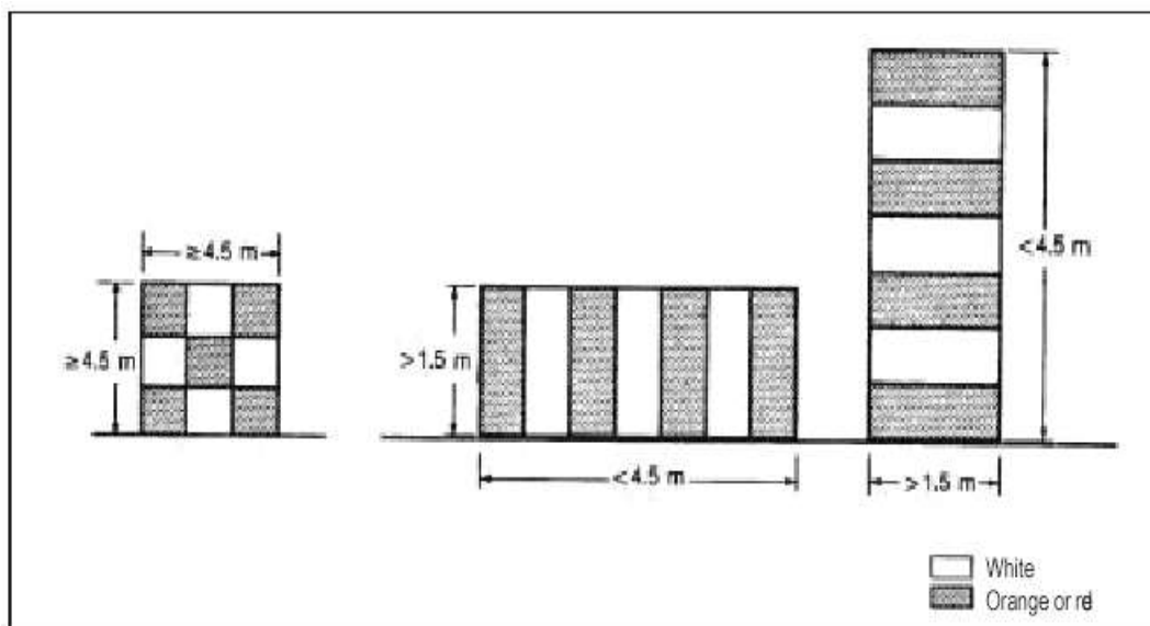
<그림 7-1> 장애물 표지의 기본형태
