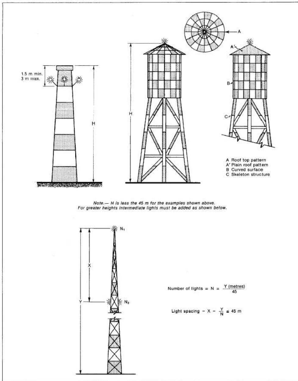
<그림 7-2> 높은 구조물의 조명과 장애물 표시의 예
